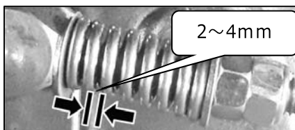
ブレーキバネの遊び (隙間)
