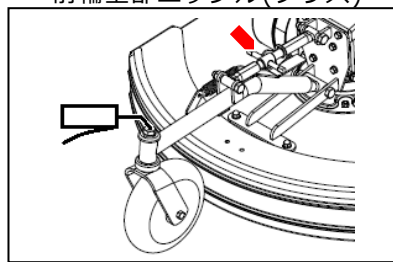
前輪上部ニップル(グリス)
