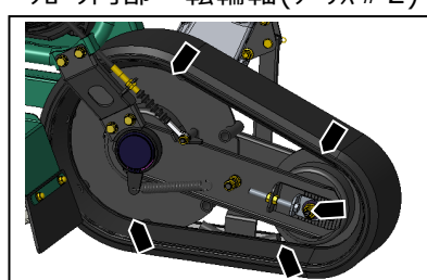
カマ内部・転輪軸(グリス #2)
