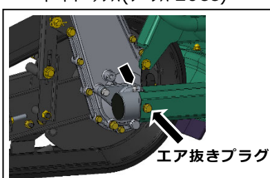
ギヤボックス(グリス 20cc)
