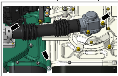
ナイフカッター結合部 ギヤボックス(グリス 30cc)
