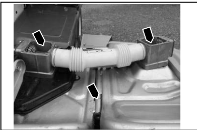
ナイフカバー結合部・ギヤボックス(グリス 40cc)
