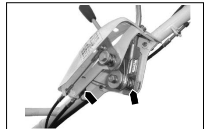
ウイング角度調整ワイヤ・レバー支点
