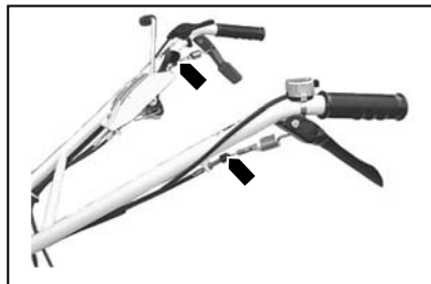
走行・ナイフクラッチワイヤ
