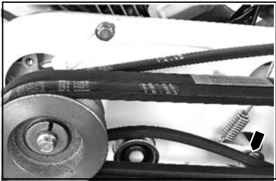
走行クラッチテンションアーム支点
